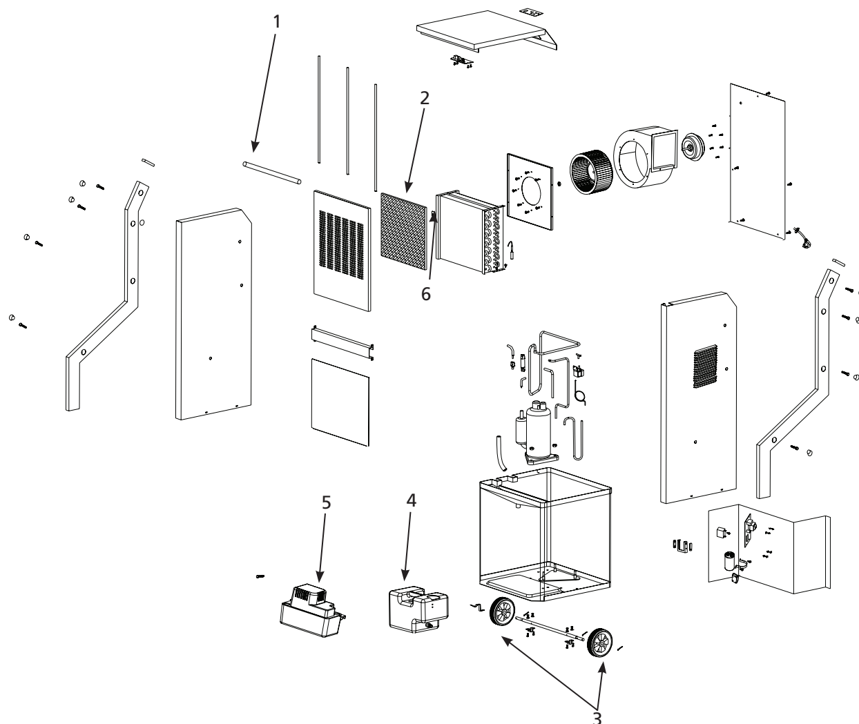
Figura 6 – Ilustración de las Partes de Reparación para los Deshumidificadores
