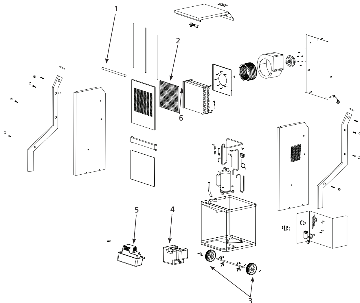
Figure 6 – Illustration des pièces détachées pour les déshumidificateurs
